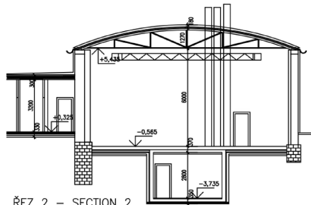
ŘEZ 2 - SECTION 2
